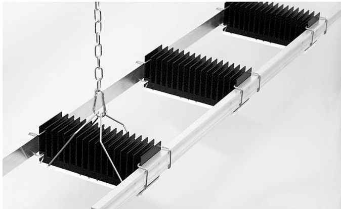
Abb. 1, fertig aufgebautes Rahmensystem
