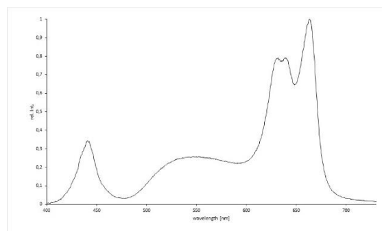
Spektrale Intensitätsverteilung
